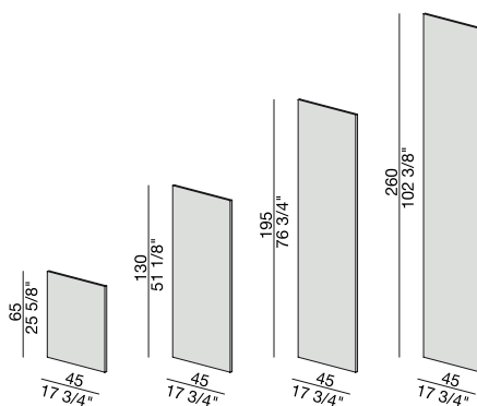
SPALLA Side
