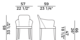
834/PI poltrona \ armchair
