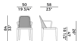
834/P poltrona \ armchair
