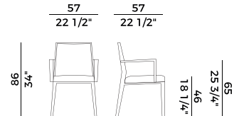
765/PII poltrona \ armchair
