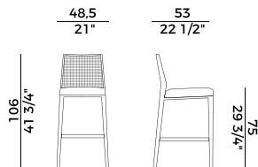
765/ACC sgabello alto \ barstool
