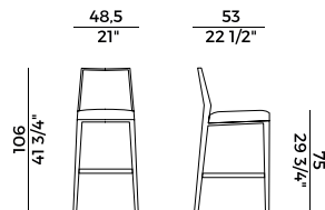
765/AII sgabello alto \ barstool
