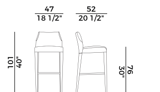
772/A sgabello alto \ barstool
