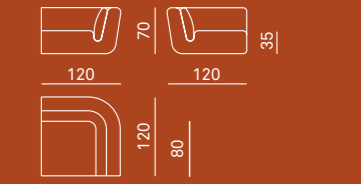
ELEMENTO ANGOLARE ANGULAR MODULE
