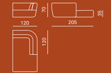
ELEMENTO ANGOLARE ANGULAR MODULE
